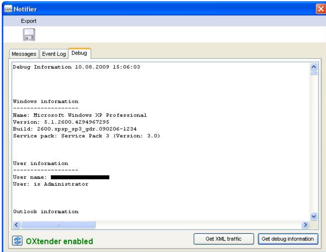
Figure 9.1. OXNotifier - Débogage
