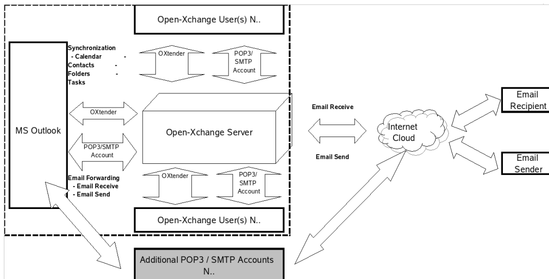
Figuur 9.5. Gebruiksmodel met gecombineerd Peer-to-Peer/Client-Server - OXtender/POP3
